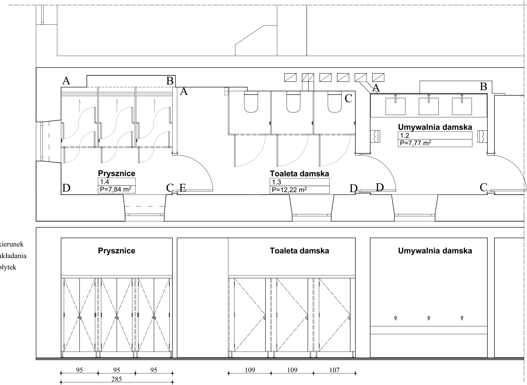
RZUT I PIĘTRA - UMYWALNIE, TOALETY I PRYSZNICE DAMSKIE SKALA 1:50
