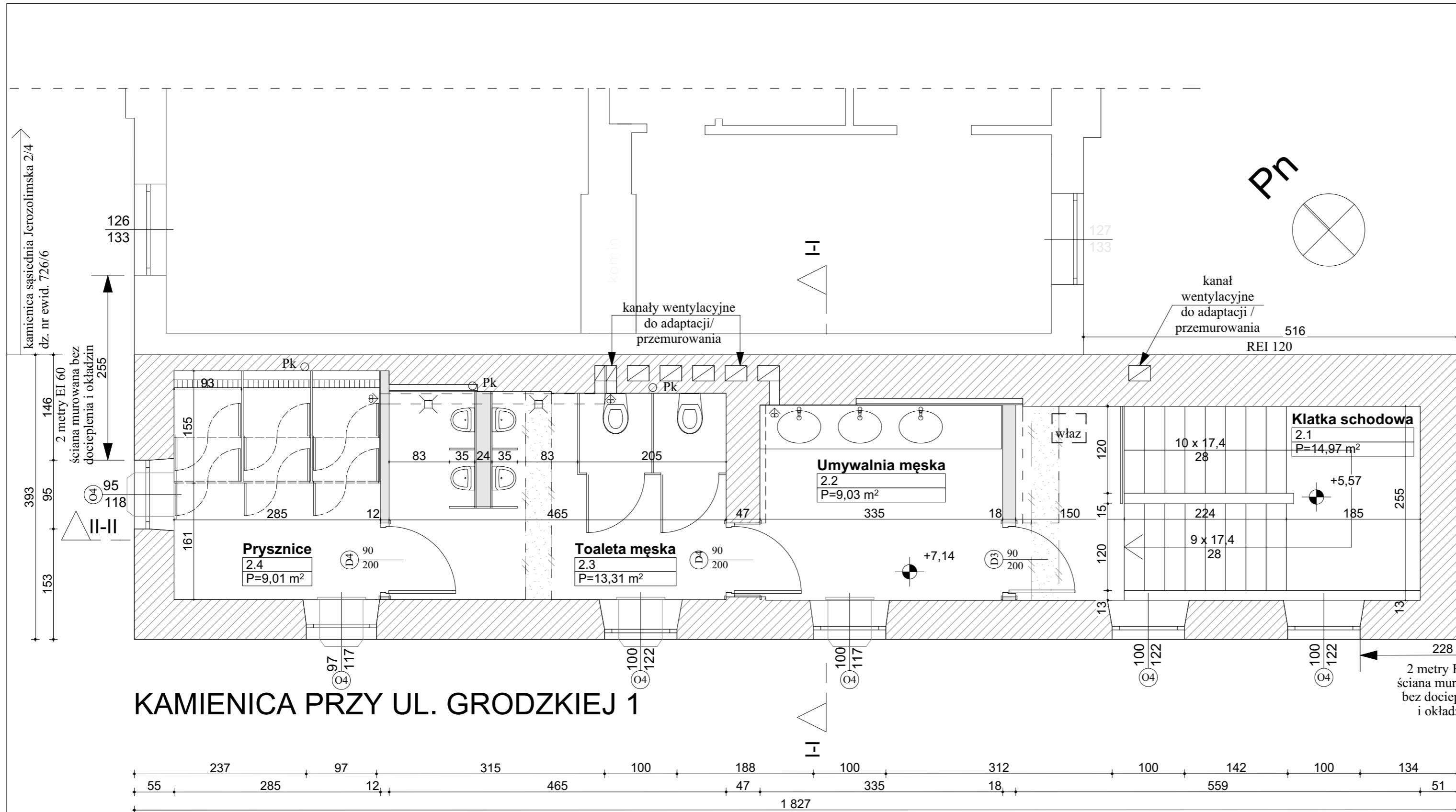
RZUT II PIĘTRA - UMYWALNIE, TOALETY I PRYSZNICE MĘSKIE SKALA 1:50
